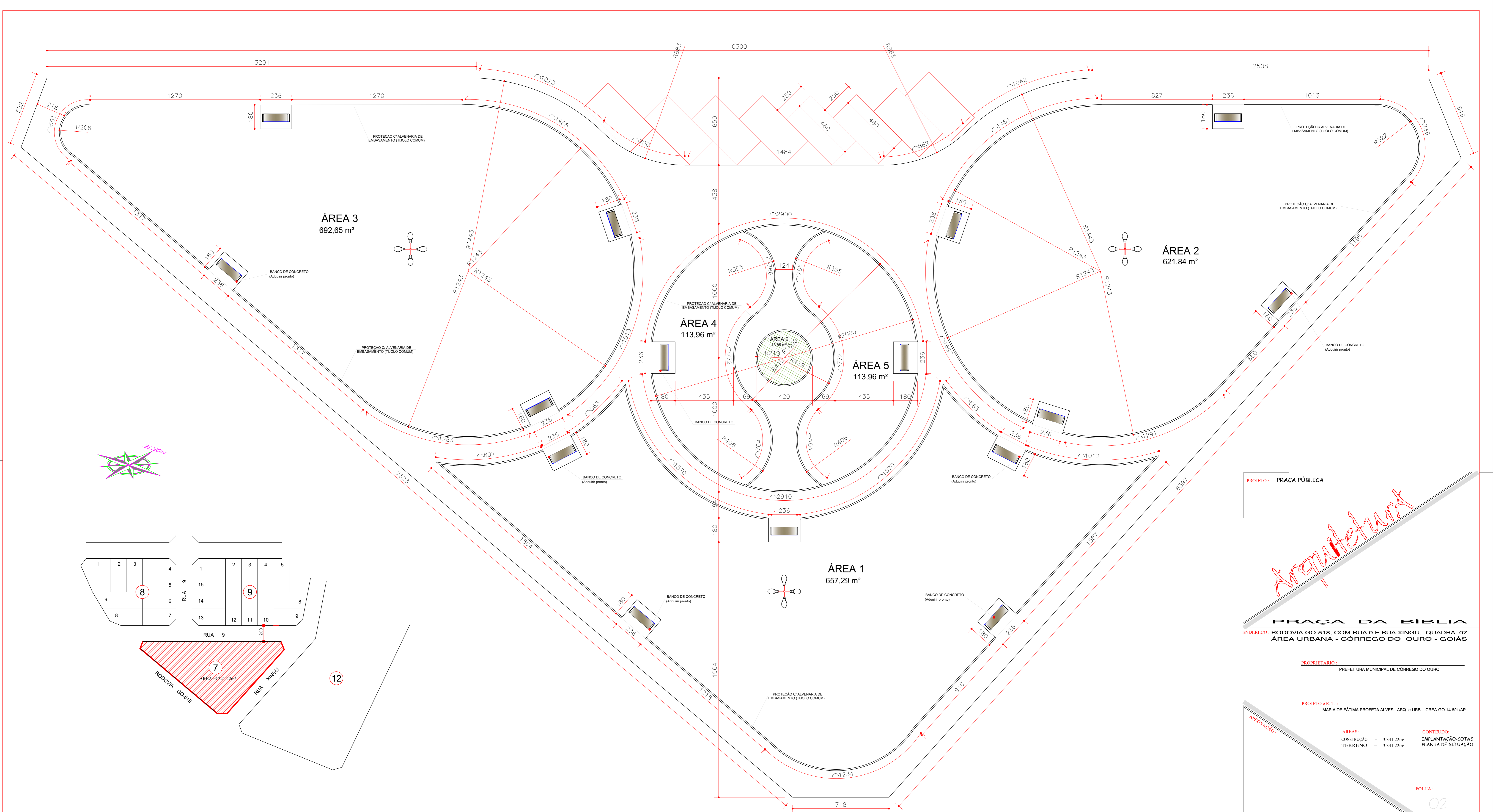
Planta de Situação Escala 1:1000
